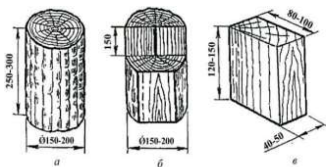
Рис.2. Образцы древесины:
