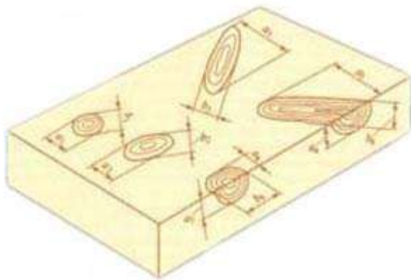
Рис.3 Измерение сучков в пиломатериале и строганом шпоне
