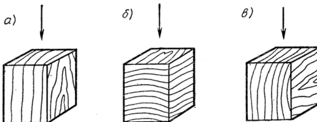
Рис. 1. Испытание механических свойств древесины на сжатие:
