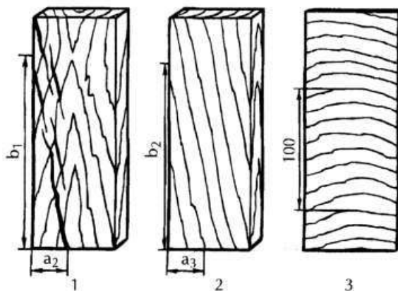
Рис.2 Измерение наклона волокон
