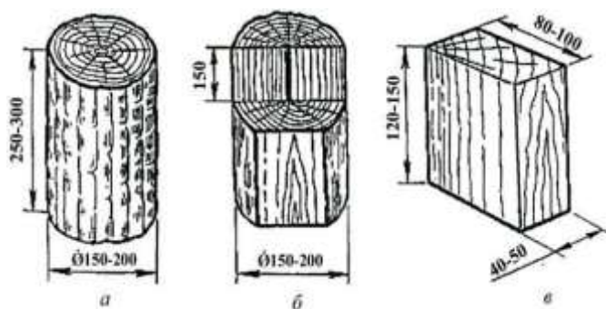
Рис.2. Образцы древесины:
