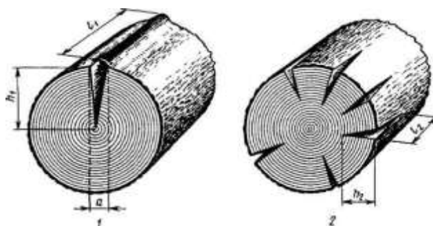
Рис.3 Измерение торцовых трещин
