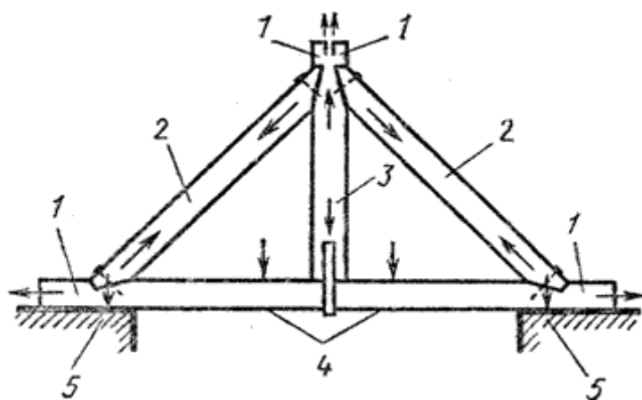
Рис.5. Направление сил в деревянной конструкции, находящейся под нагрузкой:
