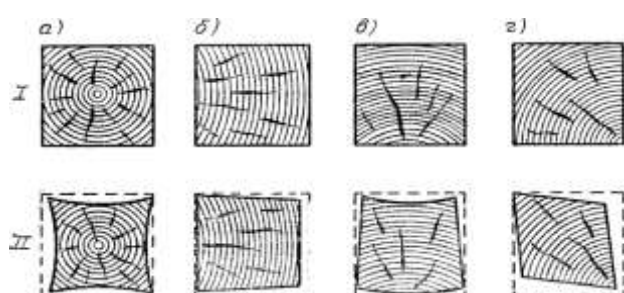
Рис. 3. Усушка и коробление граней: I — грани древесины, не подвергавшиеся сушке; II — грани высушенной древесины; а, б, в, г — схемы усушки граней древесины в зависимости от их места в стволе.
