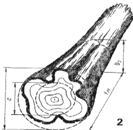
Рис.2 Закомелистость ребристая
