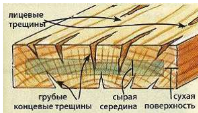
Рис.2 Виды трещин
