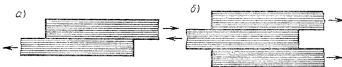
Рис.3. Сдвиг древесины: а—вдоль волокон; б—перпендикулярно волокнам.
