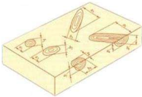
Рис.3 Измерение сучков в пиломатериале и строганом шпоне
