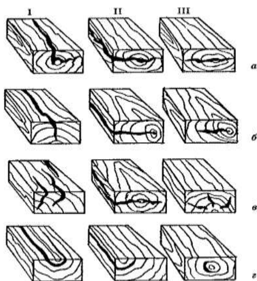
Рис.1 Типы трещин в древесине:
