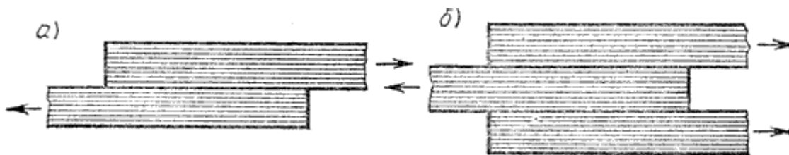
Рис.3.Сдвиг древесины: а—вдоль волокон; б—перпендикулярно волокнам.
