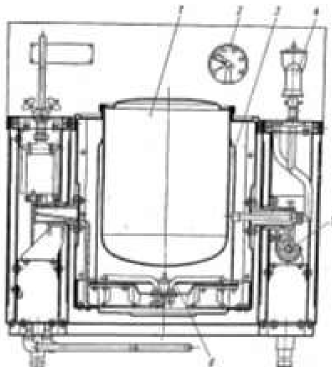
Рисунок 2 – Котел пищеварочный КПЭСМ – 60
